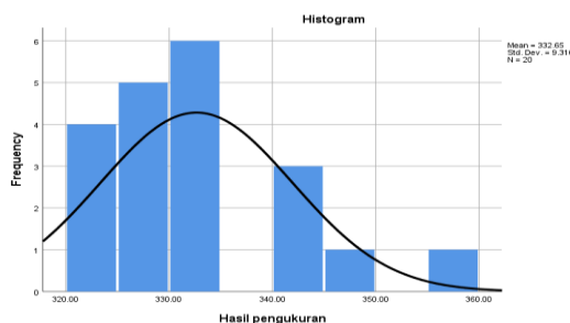
Gambar 1 Histogram dari data kuat tekan
