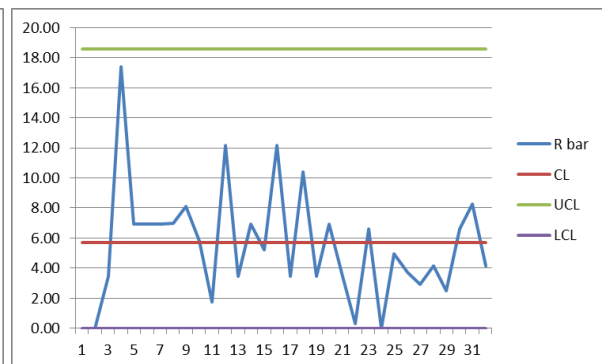
Gambar 9 Bagan Kendali R
