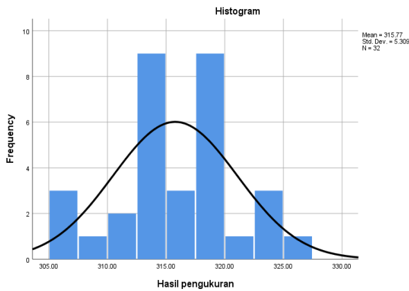
Gambar 6 Histogram dari data kuat tekan
