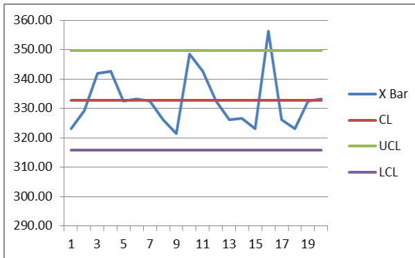
Gambar 3 Bagan Kendali X
