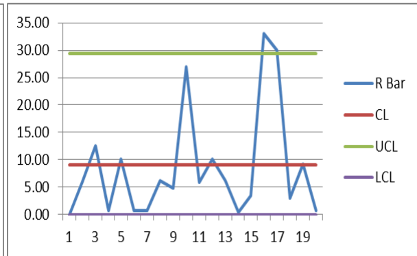
Gambar 4 Bagan Kendali R
