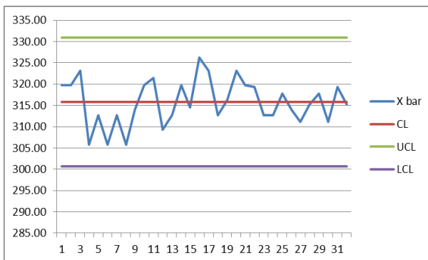
Gambar 8 Bagan Kendali X
